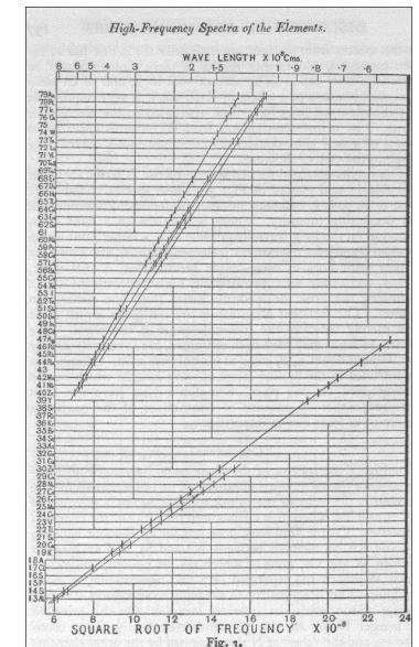
Diagramma pubblicato da Mosley nel 1914.
