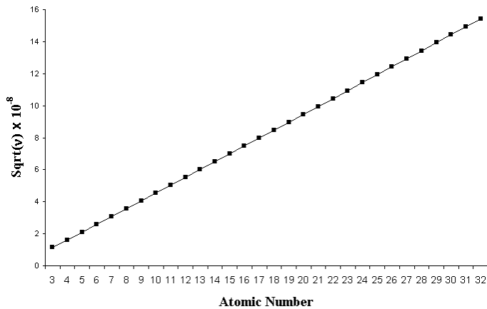
Diagramma della relazione di Mosley fra numero atomico e frequenza dei raggi X emessi da ciascun elemento
